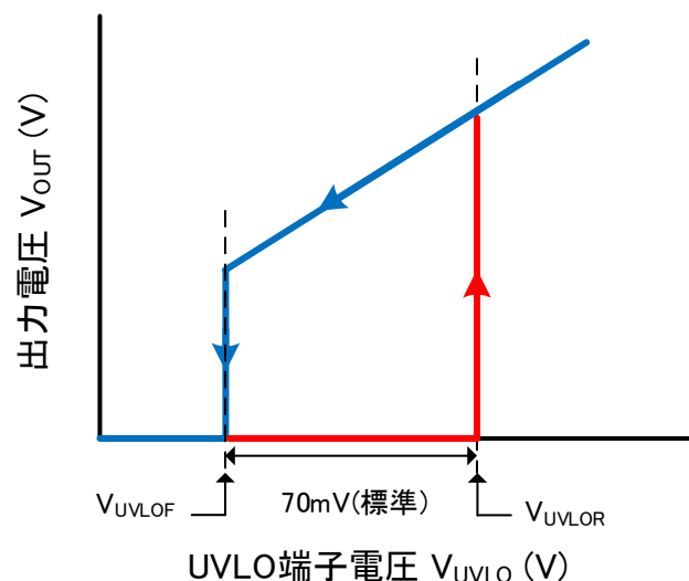
図 5.7 UVLO 検出例
