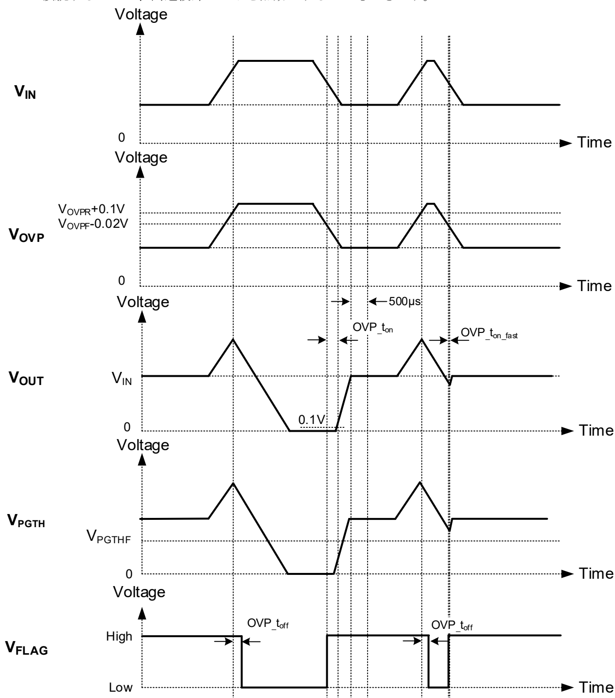
図 5.13 OVP 動作例
