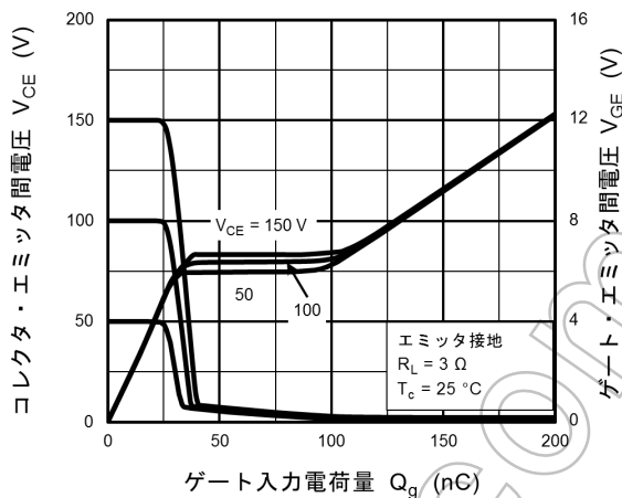
図 8.9 V_{CE}, V_{GE} - Q_g
