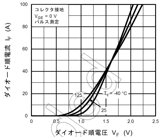
図 8.14 I_F - V_F
