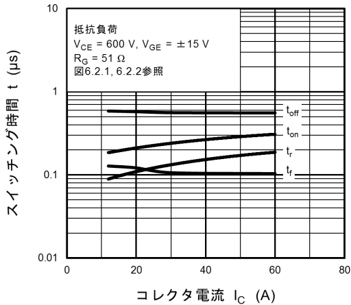
図 8.7 スイッチング時間 - I_C
