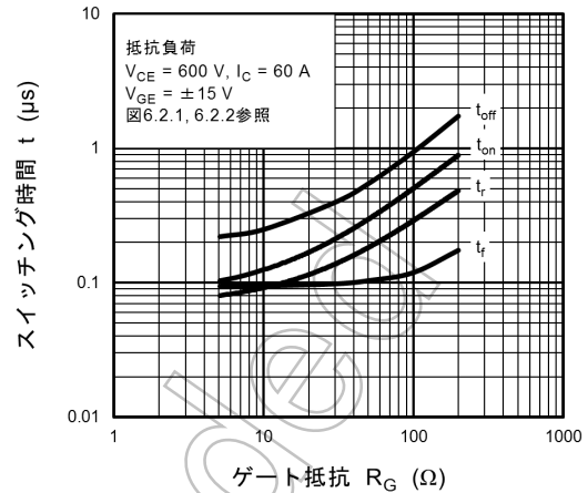
図 8.8 スイッチング時間 - R_G
