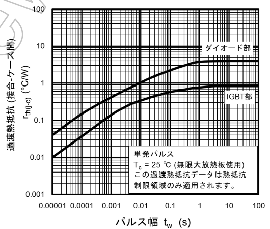
図 8.12 r_{th(j-c)} - t_w (最大値 (保証値))
