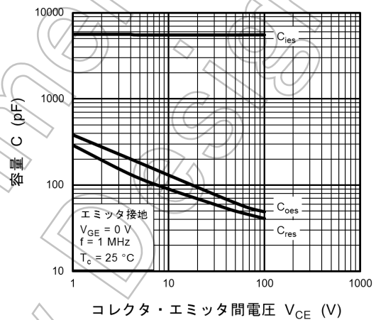
図 8.10 C - V_{CE}
