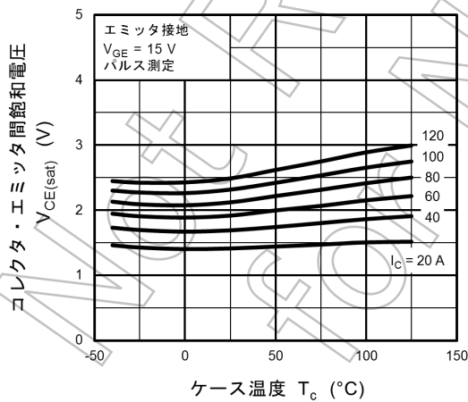
図 8.5 V_{CE(sat)} - T_c
