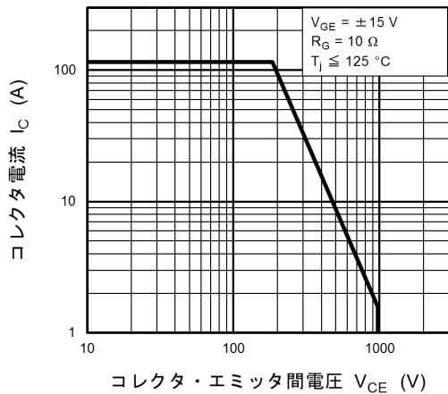
図 8.13 逆バイアス安全動作領域 (最大値 (保証値))
