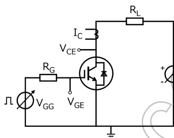
図 6.2.1 スwitchング時間の測定回路
