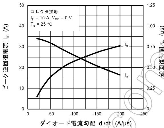
図 8.15 I_{rr}, t_{rr} - di/dt
