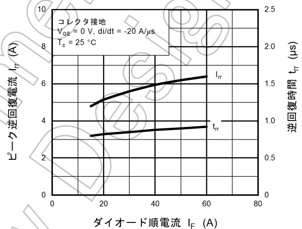
図 8.16 I_{rr}, t_{rr} - I_F
