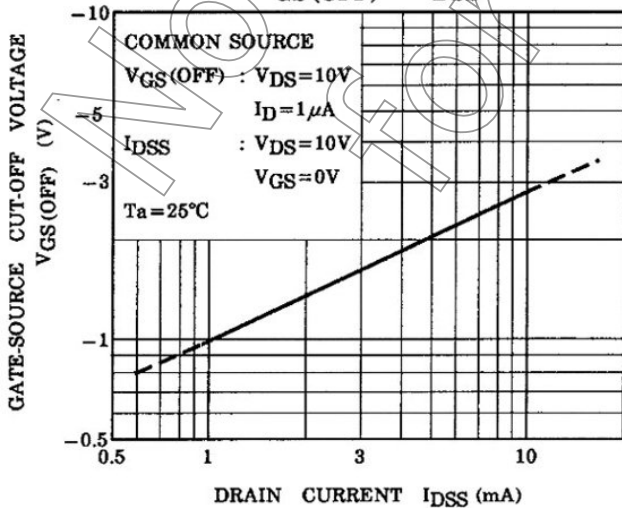
V_{GS(OFF)} - I_{DSS}
