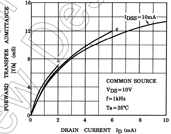
|Y_{fs}| - I_D
