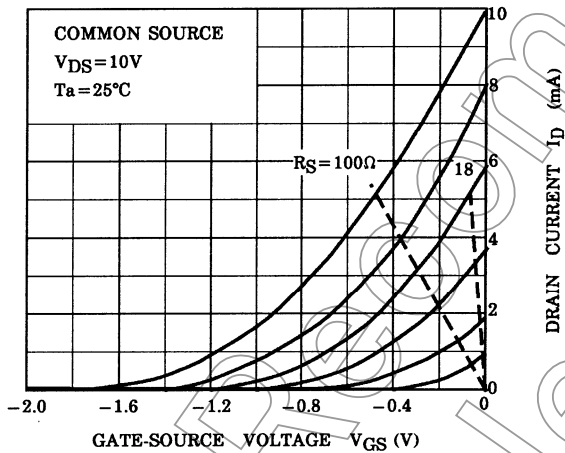
I_D - V_{GS}
