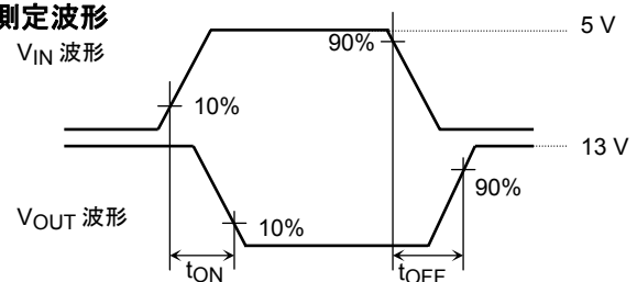
測定波形
