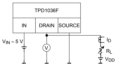
測定回路
