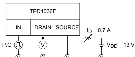
測定回路
