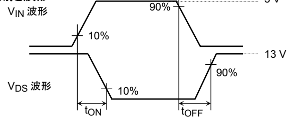
測定波形
