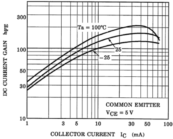
Fig. 10.15 RN1103 h_{FE}-I_C
