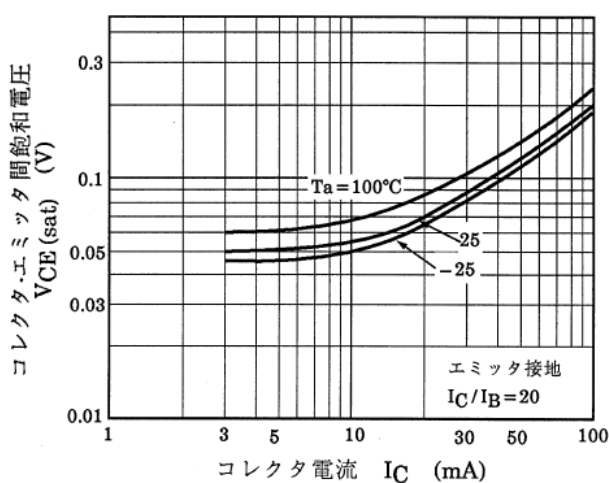
図 10.10 RN1107 V_{CE(sat)} - I_C
