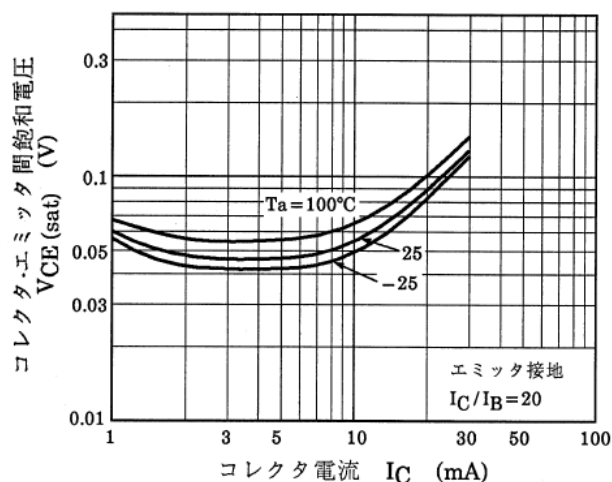
図 10.12 RN1109 V_{CE(sat)} - I_C
