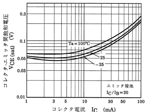
図 10.11 RN1108 V_{CE(sat)} - I_C
