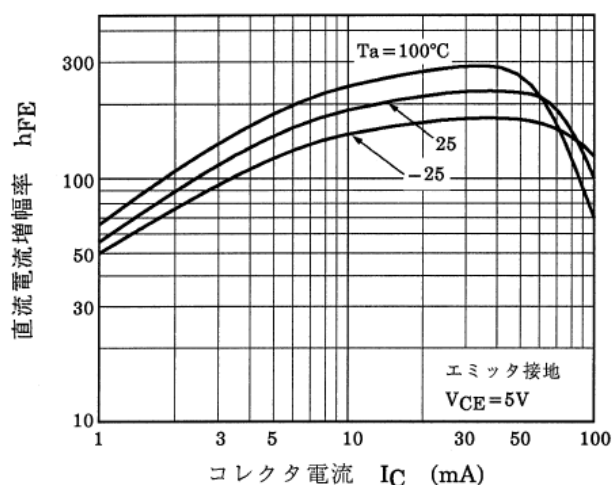
図 10.7 RN1107 h_{FE} - I_C
