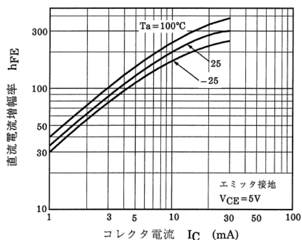
図 10.9 RN1109 h_{FE} - I_C
