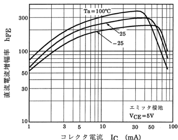
図 10.8 RN1108 h_{FE} - I_C
