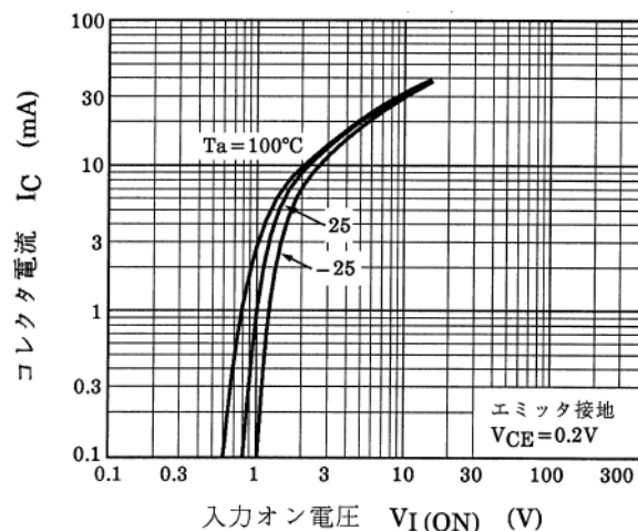
図 10.2 RN1108 I_C - V_{I(ON)}
