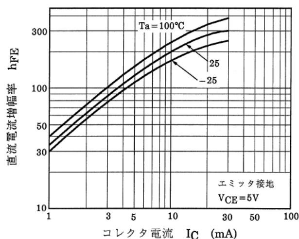
図 10.9 RN1109 h_{FE}-I_C
