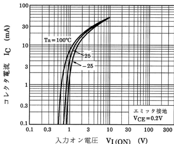
図 10.1 RN1107 I_C - V_{I(ON)}
