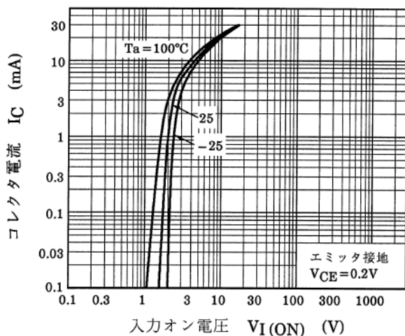
図 10.3 RN1109 I_C - V_{I(ON)}
