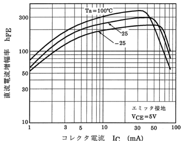
図 10.8 RN1108 h_{FE}-I_C
