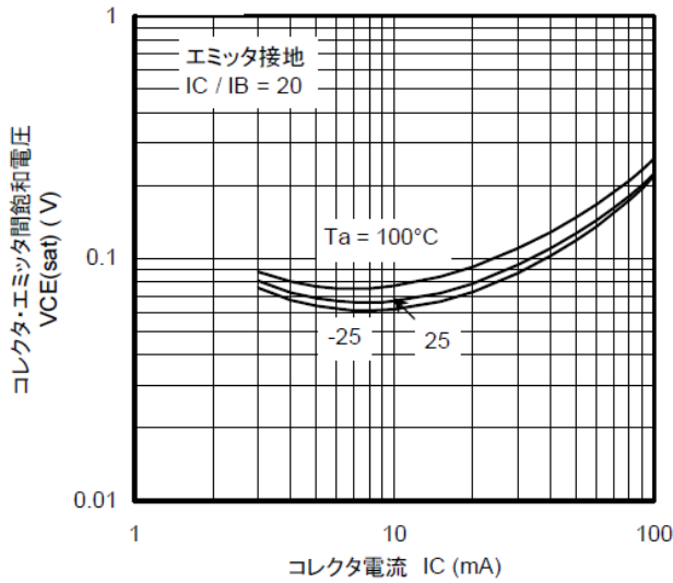
図 10.16 RN1114 V_{CE(sat)}-I_C
