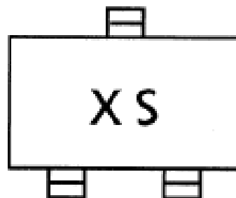
图 9.2 現品表示 RN1115
