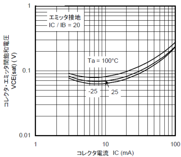
図 10.18 RN1116 V_{CE(sat)}-I_C
