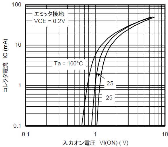
図 10.3 RN1116 I_C - V_{I(ON)}
