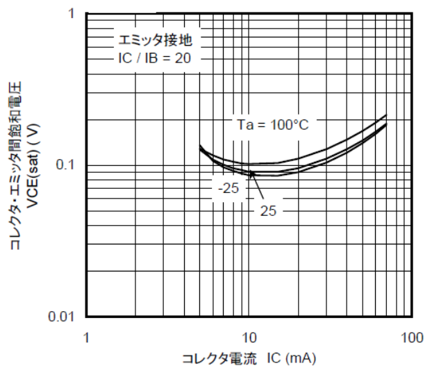
図 10.19 RN1117 V_{CE(sat)}-I_C
