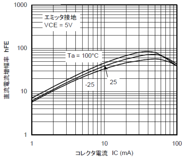
図 10.14 RN1117 h_{FE}-I_C
