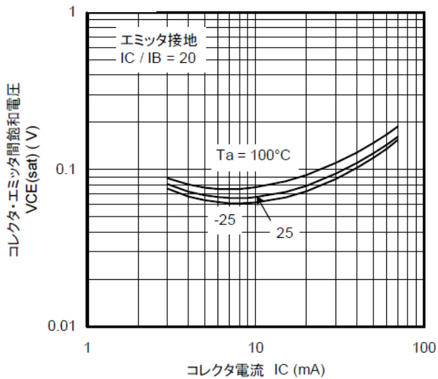
図 10.20 RN1118 V_{CE(sat)}-I_C
