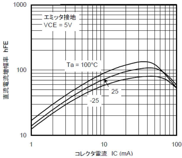
図 10.11 RN1114 h_{FE}-I_C
