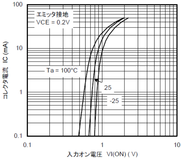
図 10.1 RN1114 I_C - V_{I(ON)}
