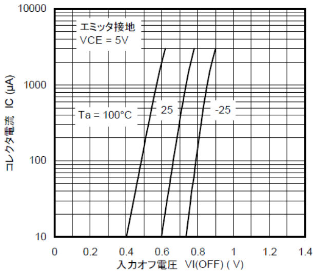
図 10.6 RN1114 I_C - V_{I(OFF)}
