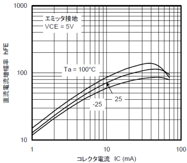
図 10.13 RN1116 h_{FE}-I_C
