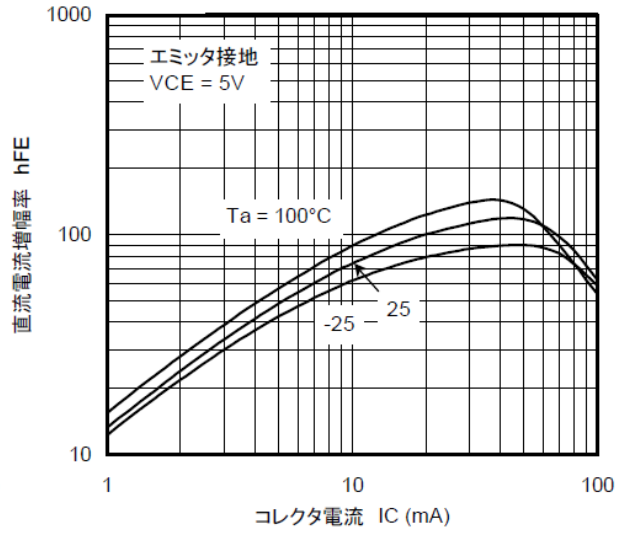
図 10.12 RN1115 h_{FE}-I_C
