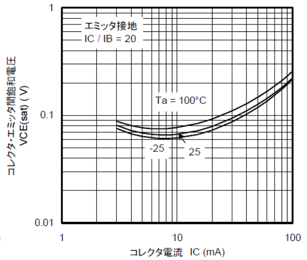
図 10.17 RN1115 V_{CE(sat)}-I_C
