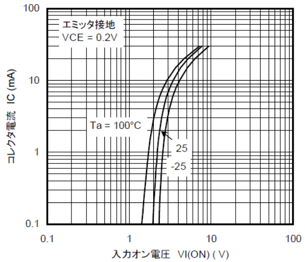
図 10.4 RN1117 I_C - V_{I(ON)}
