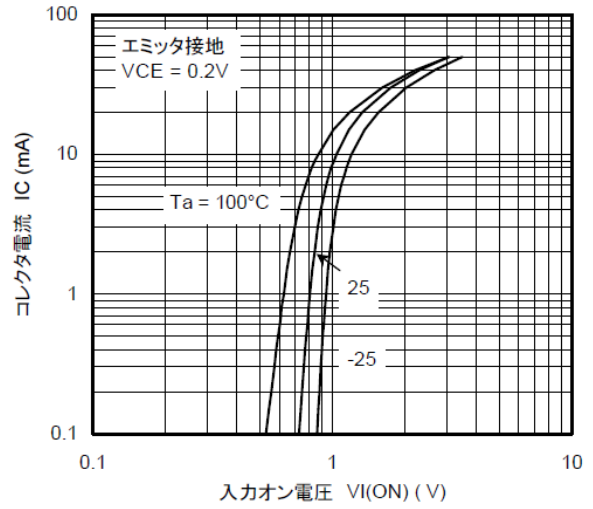
図 10.2 RN1115 I_C - V_{I(ON)}
