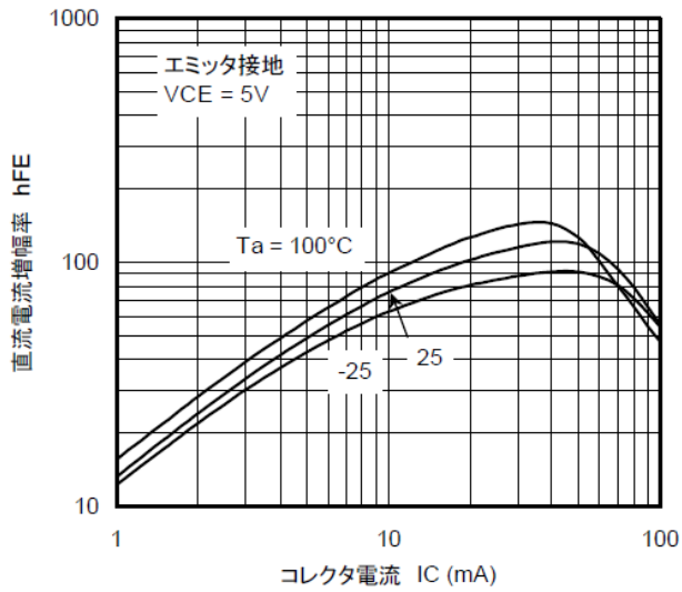
図 10.13 RN1116 h_{FE}-I_C
