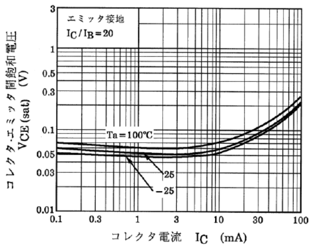
図 9.7 RN1310 V_{CE(sat)}-I_C
