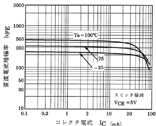
図 9.6 RN1311 h_{FE} - I_C
