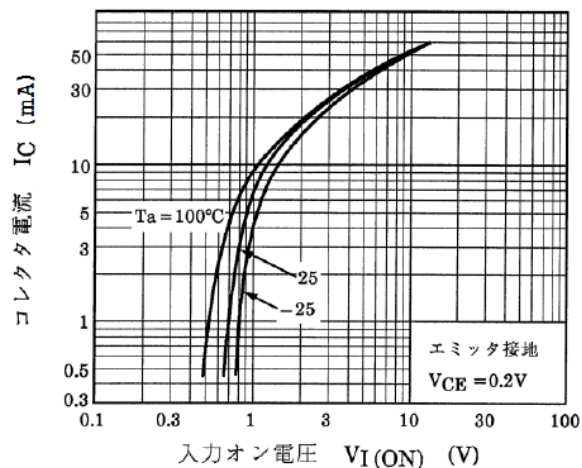
図 9.2 RN1311 I_C - V_{I(ON)}
