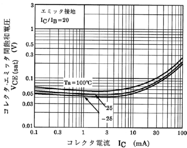
図 9.8 RN1311 V_{CE(sat)}-I_C
