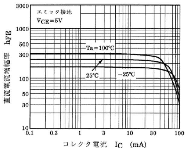
図 9.5 RN1312 h_{FE} - I_C
