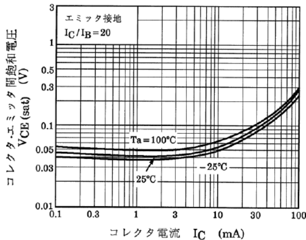
図 9.8 RN1313 V_{CE(sat)}-I_C
