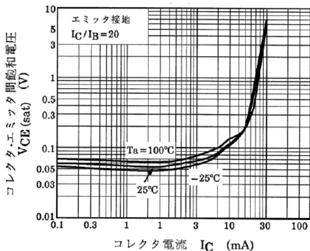
図 9.7 RN1312 V_{CE(sat)}-I_C
