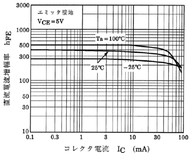
図 9.6 RN1313 h_{FE} - I_C
