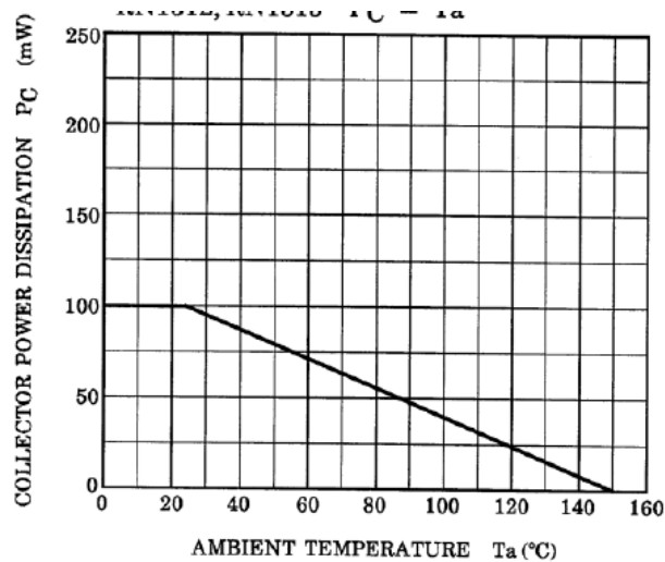
Fig. 9.9 RN1312,RN1313 P_C-T_a
