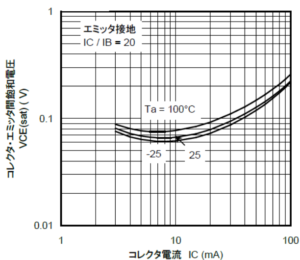
図 9.16 RN1314 V_{CE(sat)} - I_C
