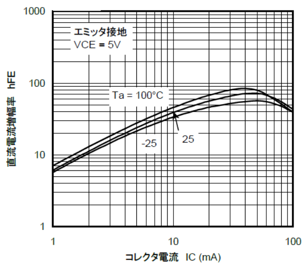
図 9.14 RN1317 h_{FE} - I_C
