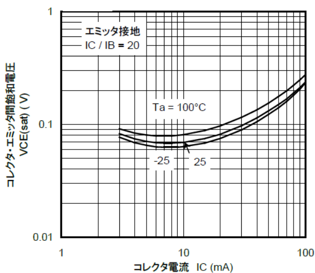
図 9.18 RN1316 V_{CE(sat)} - I_C
