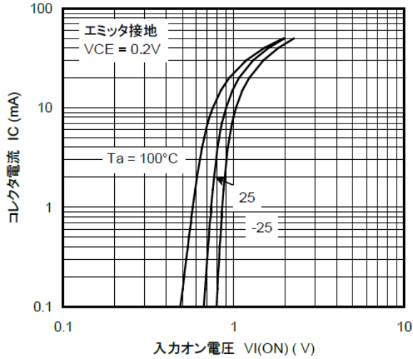
図 9.1 RN1314 I_C - V_{I(ON)}
