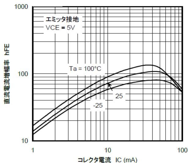
図 9.11 RN1314 h_{FE} - I_C
