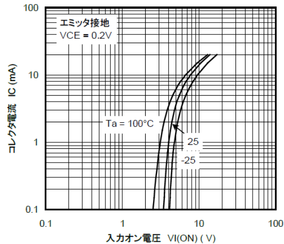
図 9.3 RN1316 I_C - V_{I(ON)}
