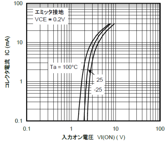
図 9.4 RN1317 I_C - V_{I(ON)}
