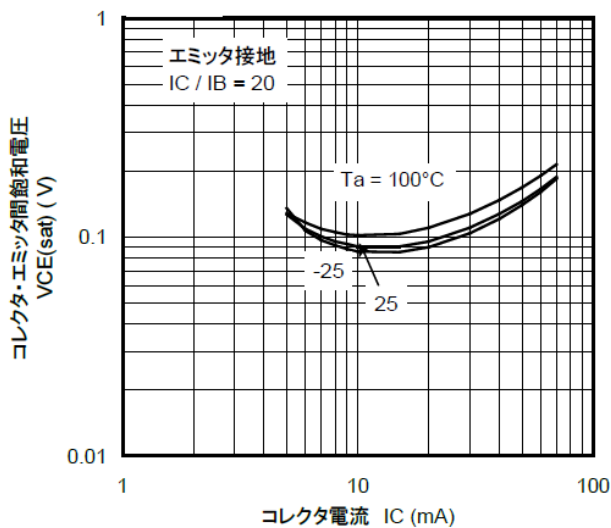
図 9.19 RN1317 V_{CE(sat)}-I_C
