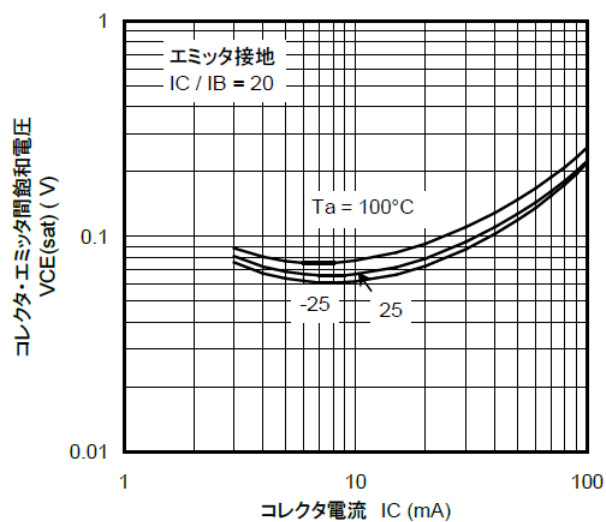
図 9.17 RN1315 V_{CE(sat)} - I_C
