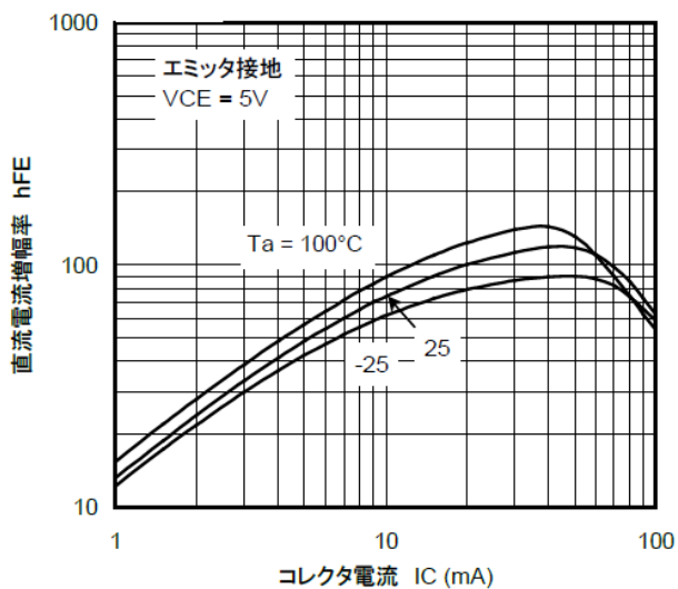
図 9.12 RN1315 h_{FE} - I_C
