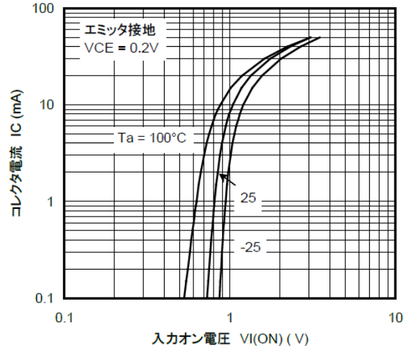
図 9.2 RN1315 I_C - V_{I(ON)}
