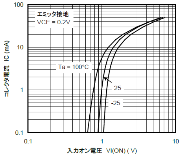
図 9.3 RN1316 I_C - V_{I(ON)}
