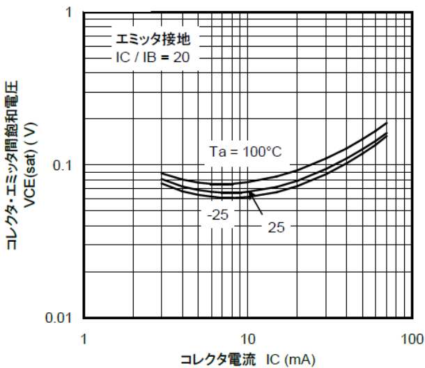
図 9.20 RN1318 V_{CE(sat)}-I_C
