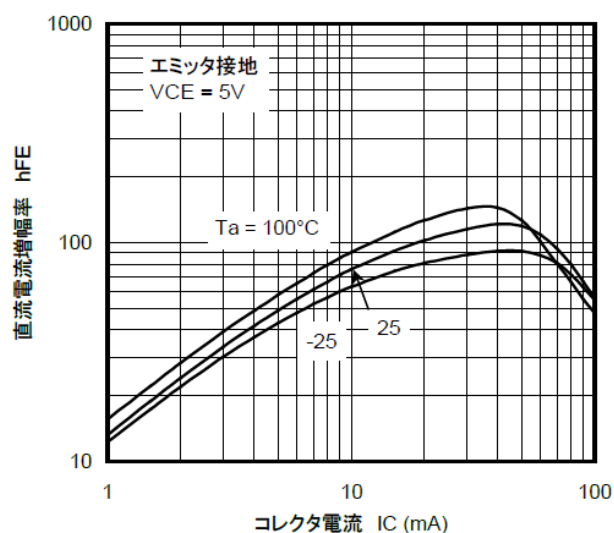
図 9.13 RN1316 h_{FE} - I_C
