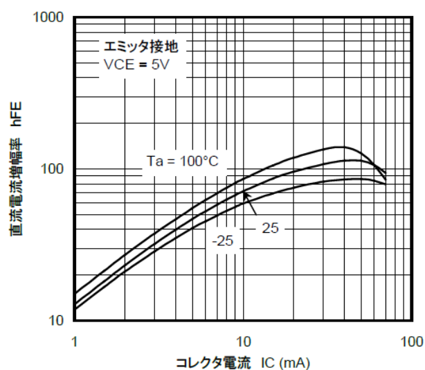
図 9.15 RN1318 h_{FE} - I_C
