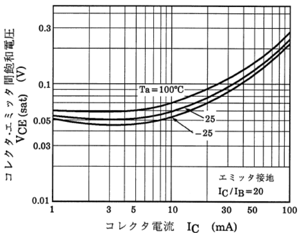
図 10.11 RN1408 V_{CE(sat)}-I_C
