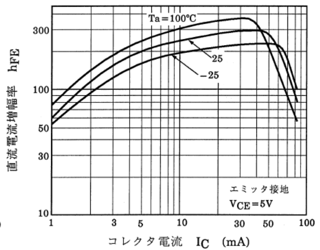
図 10.8 RN1408 h_{FE}-I_C
