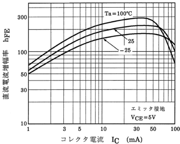
図 10.7 RN1407 h_{FE}-I_C
