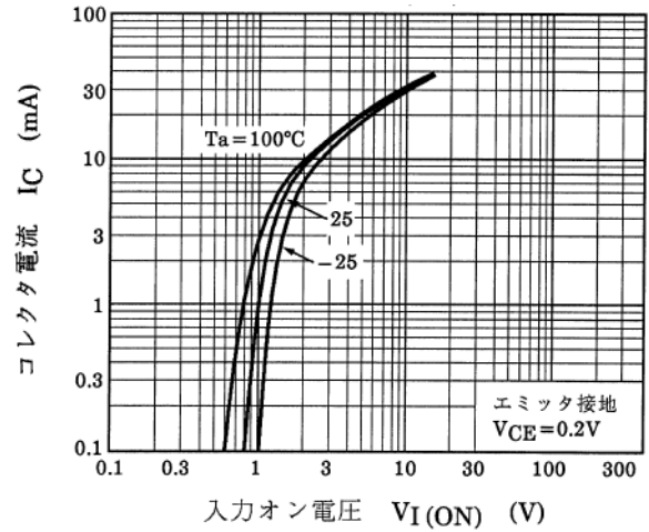
図 10.2 RN1408 I_C - V_{I(ON)}
