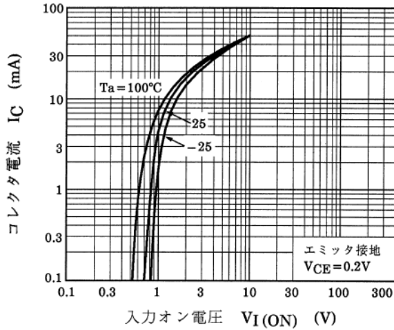
図 10.1 RN1407 I_C - V_{I(ON)}
