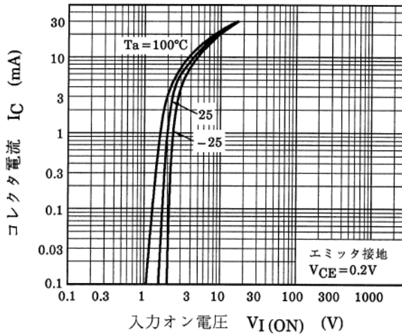
図 10.3 RN1409 I_C - V_{I(ON)}
