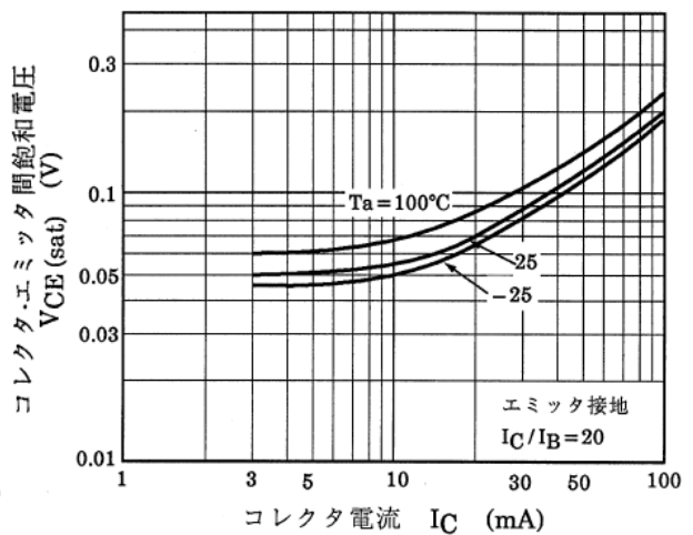
図 10.10 RN1407 V_{CE(sat)}-I_C
