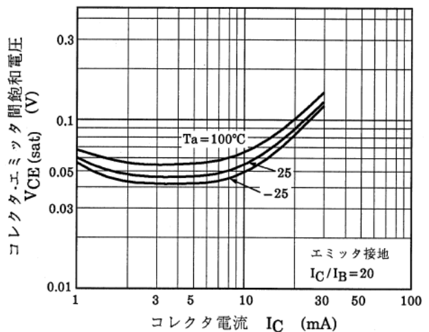
図 10.12 RN1409 V_{CE(sat)}-I_C
