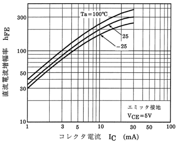
図 10.9 RN1409 h_{FE}-I_C
