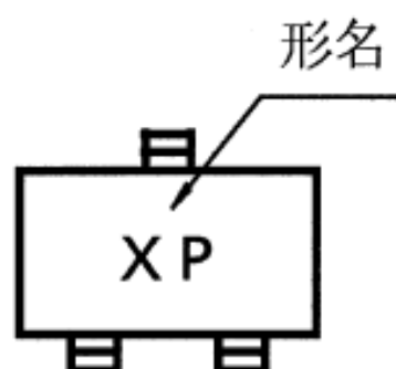
図 8.2 現品表示 RN1413
