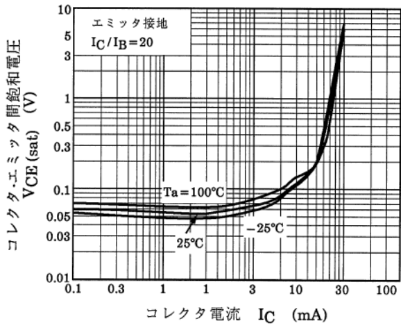
図 9.7 RN1412 V_{CE(sat)}-I_C
