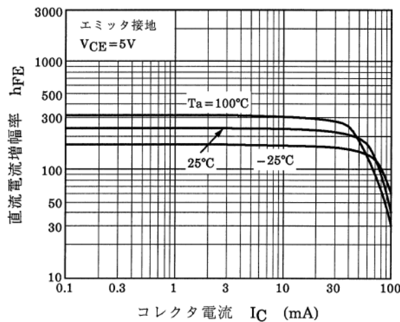
図 9.5 RN1412 h_{FE} - I_C
