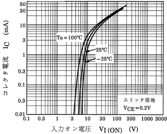
図 9.1 RN1412 I_C - V_{I(ON)}
