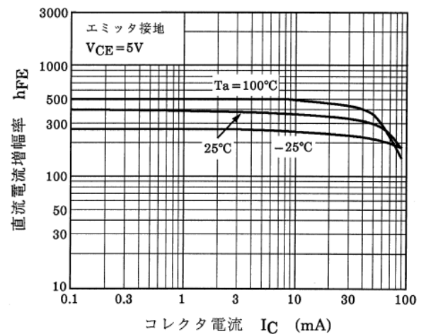
図 9.6 RN1413 h_{FE} - I_C
