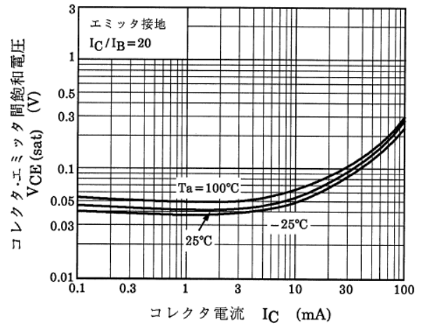
図 9.8 RN1413 V_{CE(sat)}-I_C
