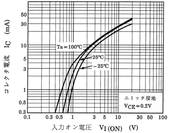
図 9.2 RN1413 I_C - V_{I(ON)}
