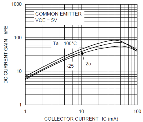
Fig. 10.14 RN1417 h_{FE} - I_C
