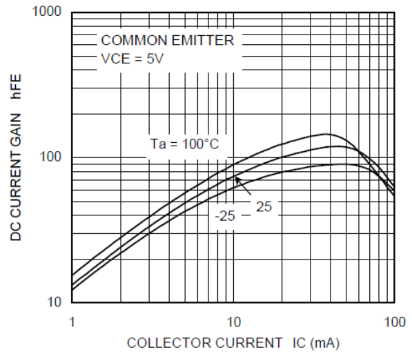
Fig. 10.12 RN1415 h_{FE} - I_C
