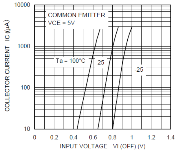
Fig. 10.7 RN1415 I_C - V_I (OFF)
