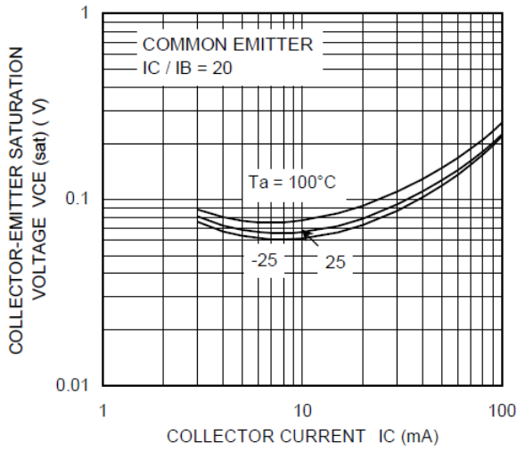
Fig. 10.16 RN1414 V_{CE(sat)} - I_C
