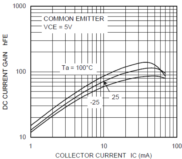
Fig. 10.13 RN1416 h_{FE} - I_C
