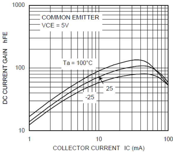
Fig. 10.11 RN1414 h_{FE} - I_C
