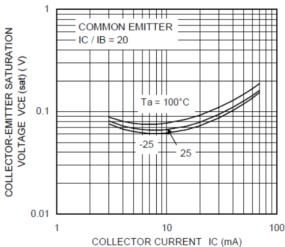
Fig. 10.18 RN1416 V_{CE(sat)} - I_C
