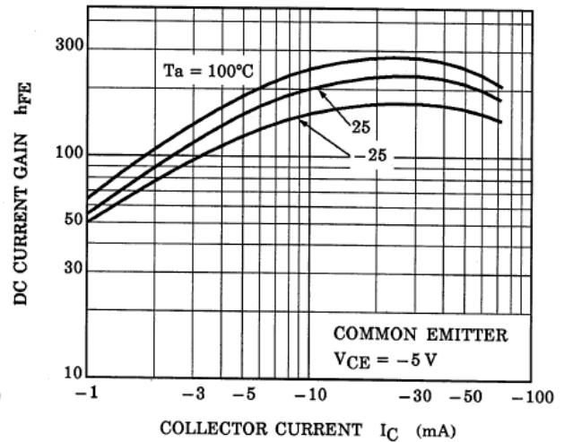
Fig. 10.16 RN2104 h_{FE} - I_C
