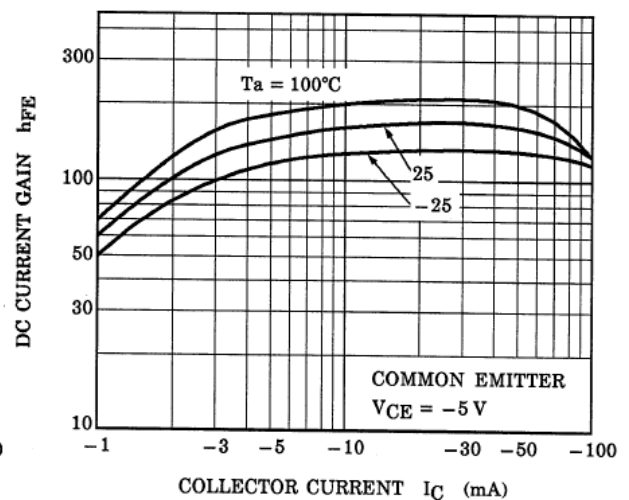
Fig. 10.18 RN2106 h_{FE} - I_C
