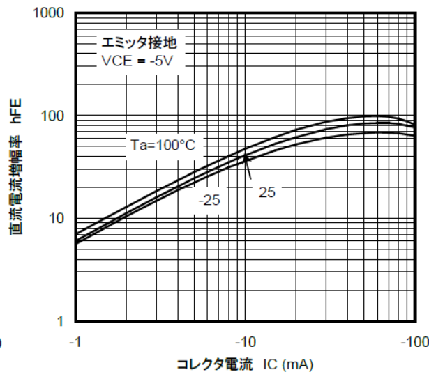
図 10.14 RN2117 h_{FE}-I_C
