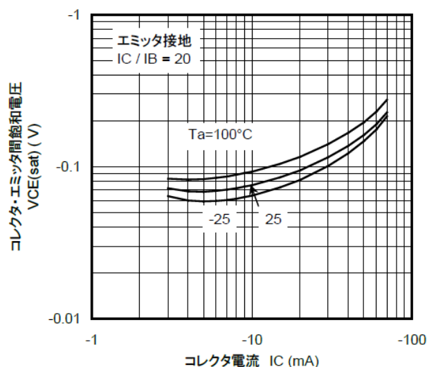
図 10.20 RN2118 V_{CE(sat)} - I_C
