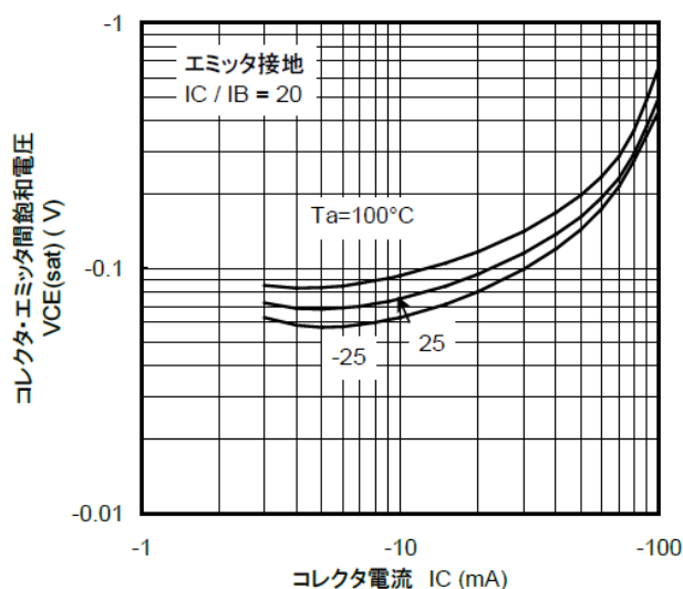
図 10.18 RN2116 V_{CE(sat)} - I_C
