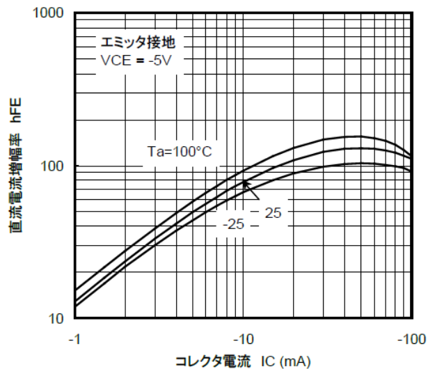
図 10.12 RN2115 h_{FE}-I_C
