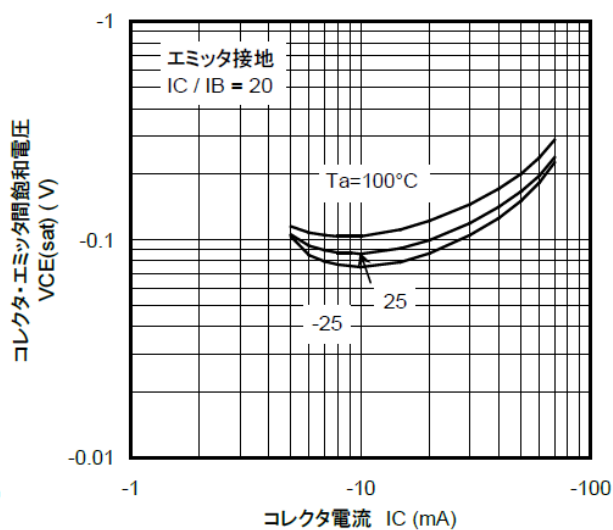
図 10.19 RN2117 V_{CE(sat)} - I_C
