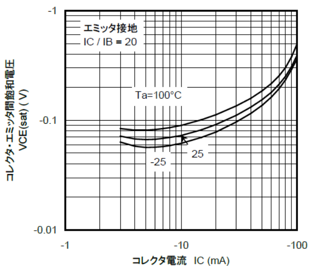
図 10.17 RN2115 V_{CE(sat)} - I_C
