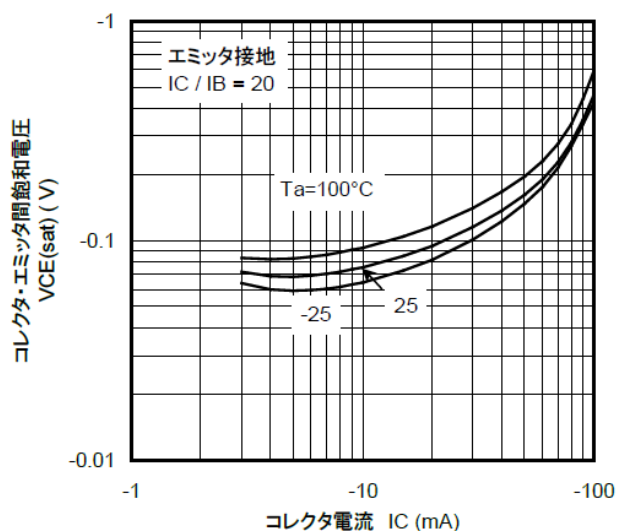
図 10.16 RN2114 V_{CE(sat)} - I_C
