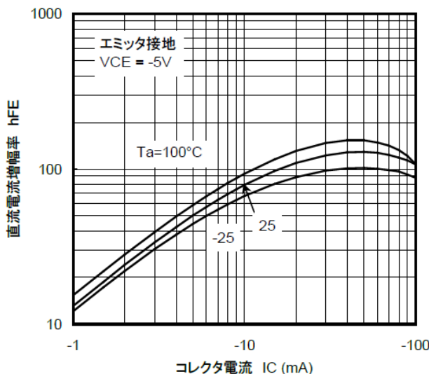
図 10.13 RN2116 h_{FE}-I_C
