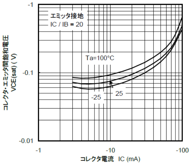
図 10.18 RN2116 V_{CE(sat)}-I_C
