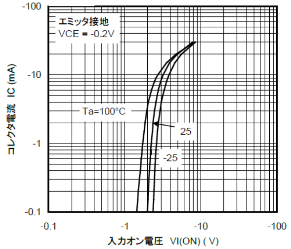
図 10.4 RN2117 I_C - V_{I(ON)}
