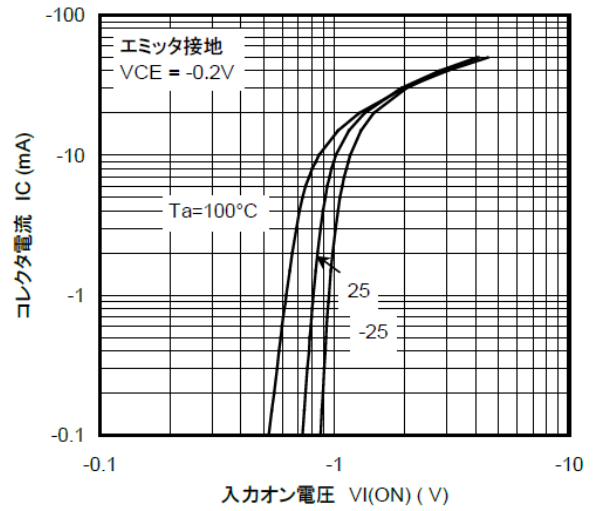
図 10.2 RN2115 I_C - V_{I(ON)}
