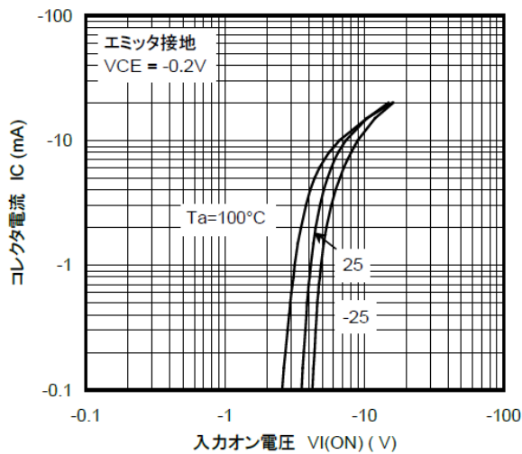
図 10.3 RN2116 I_C - V_{I(ON)}
