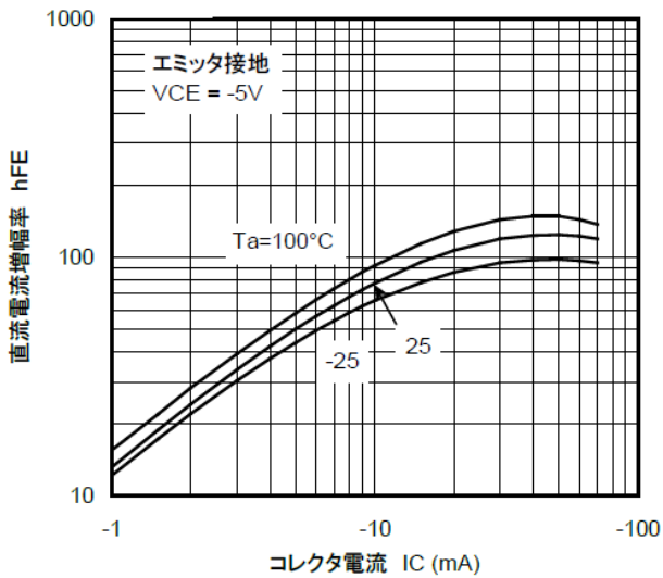
図 10.13 RN2116 h_{FE}-I_C
