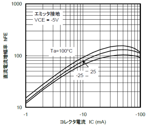
図 10.12 RN2115 h_{FE}-I_C
