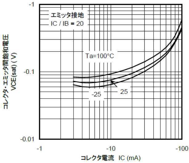
図 10.16 RN2114 V_{CE(sat)}-I_C
