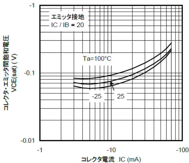
図 10.20 RN2118 V_{CE(sat)}-I_C
