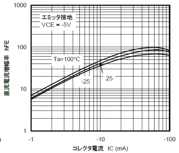
図 10.14 RN2117 h_{FE}-I_C
