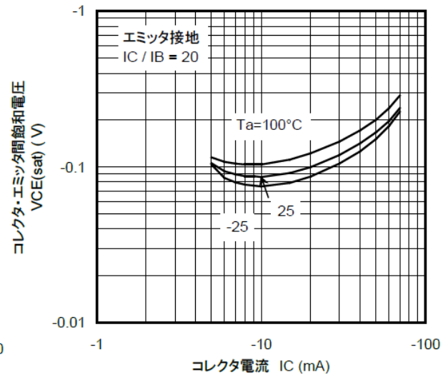
図 10.19 RN2117 V_{CE(sat)}-I_C
