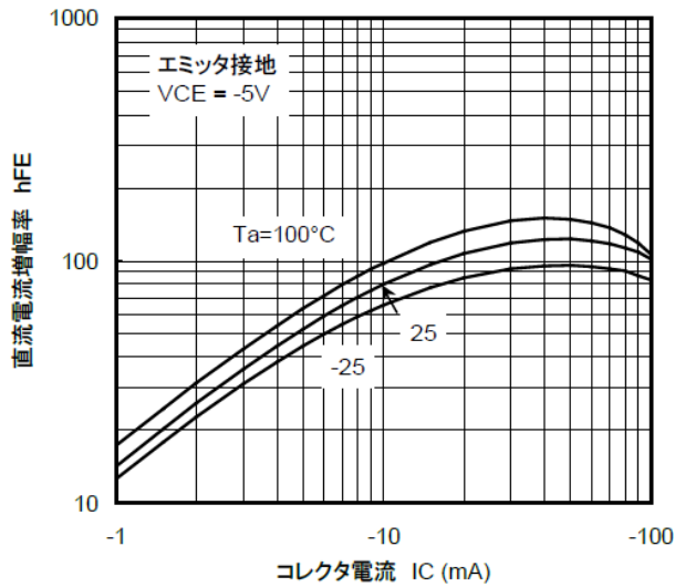
図 10.11 RN2114 h_{FE}-I_C
