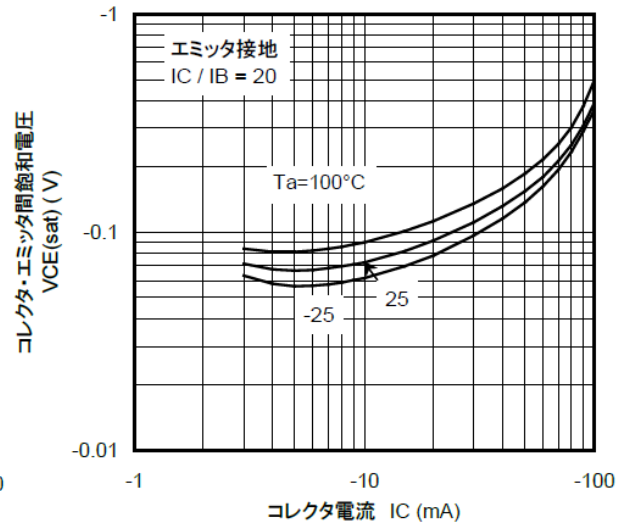
図 10.17 RN2115 V_{CE(sat)}-I_C
