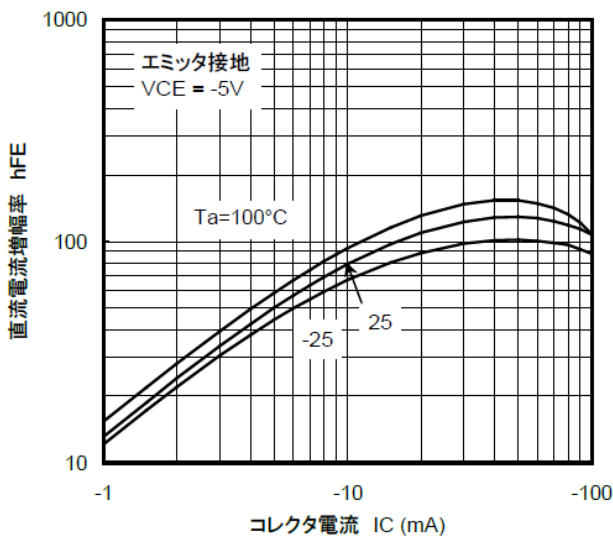
図 10.13 RN2116 h_{FE}-I_C
