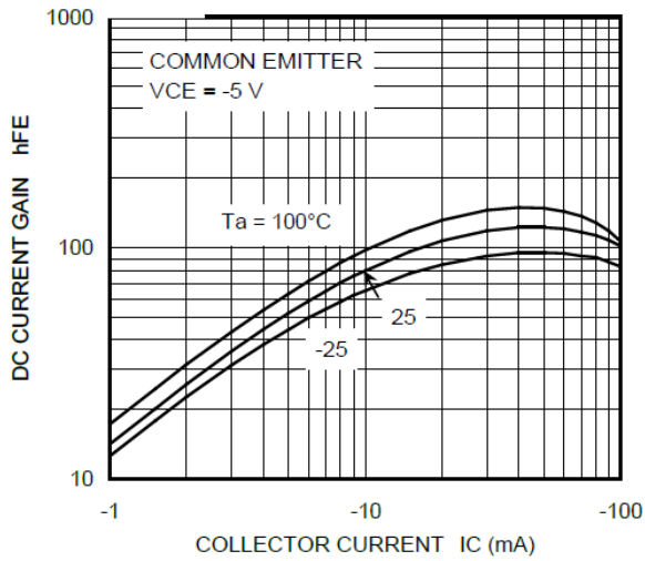
Fig. 10.11 RN2114 h_{FE}-I_C
