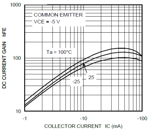
Fig. 10.13 RN2116 h_{FE}-I_C
