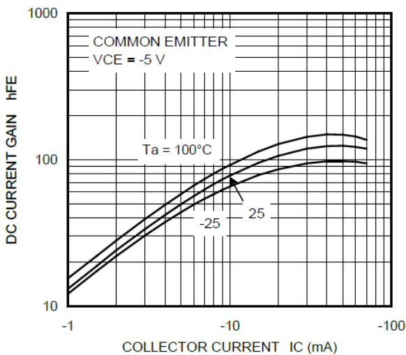
Fig. 10.13 RN2116 h_{FE}-I_C
