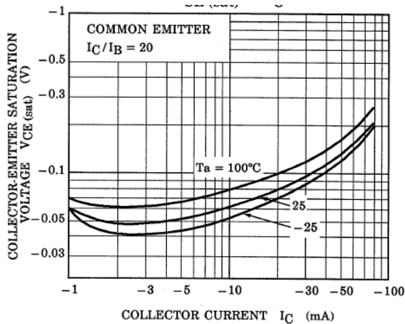
Fig. 10.21 RN2403 V_{CE(sat)} - I_C
