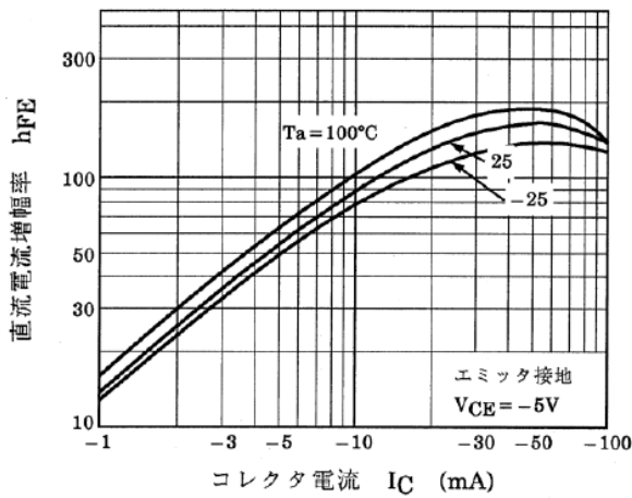
図 10.7 RN2407 h_{FE}-I_C
