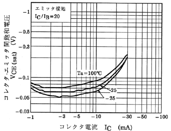
図 10.12 RN2409 V_{CE(sat)}-I_C
