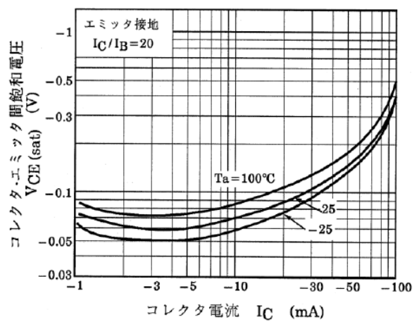
図 10.10 RN2407 V_{CE(sat)}-I_C
