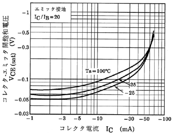
図 10.11 RN2408 V_{CE(sat)}-I_C
