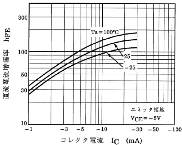
図 10.9 RN2409 h_{FE}-I_C
