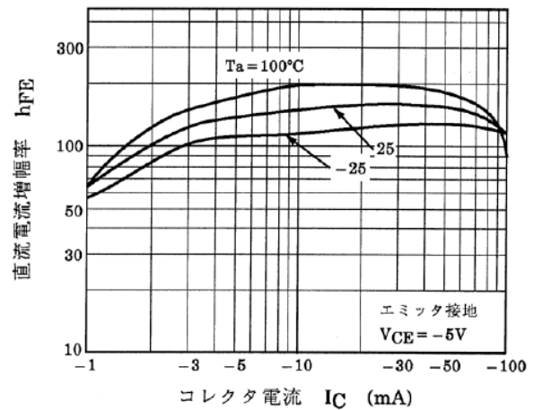
図 10.8 RN2408 h_{FE}-I_C
