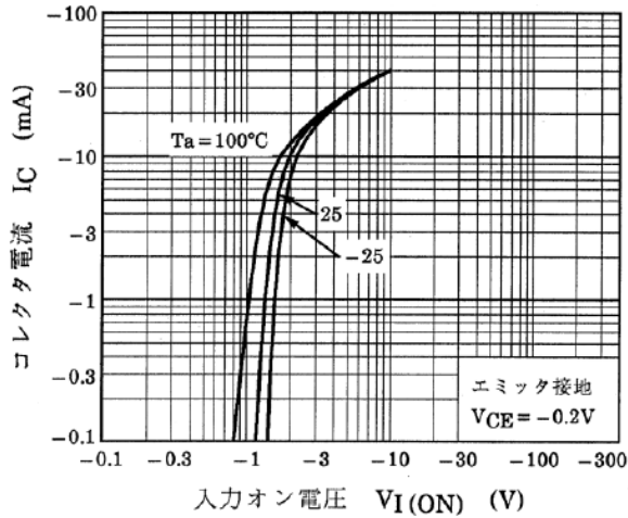
図 10.1 RN2407 I_C - V_{I(ON)}
