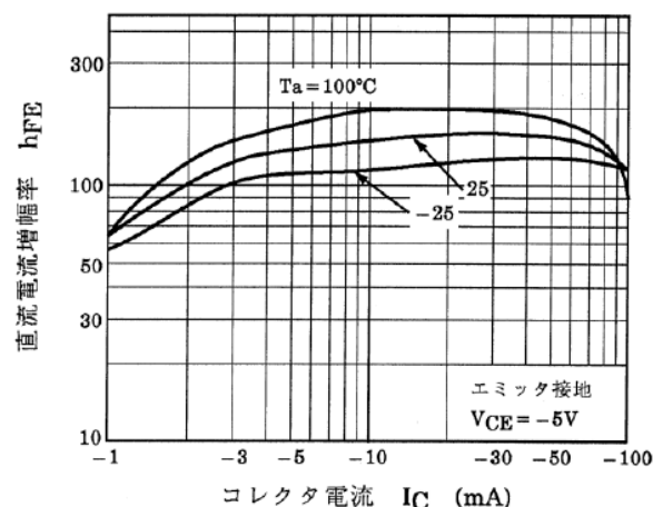
図 10.8 RN2408 h_{FE} - I_C
