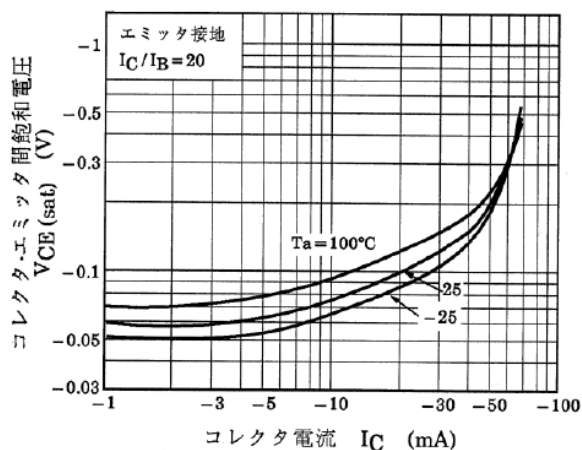
図 10.11 RN2408 V_{CE(sat)} - I_C
