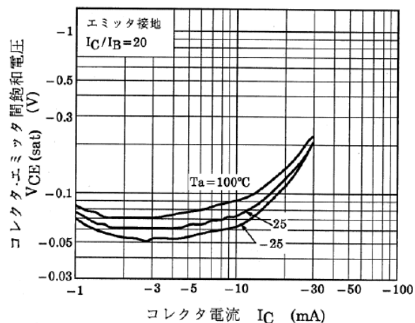
図 10.12 RN2409 V_{CE(sat)} - I_C
