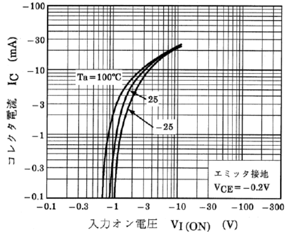
図 10.2 RN2408 I_C - V_{I(ON)}
