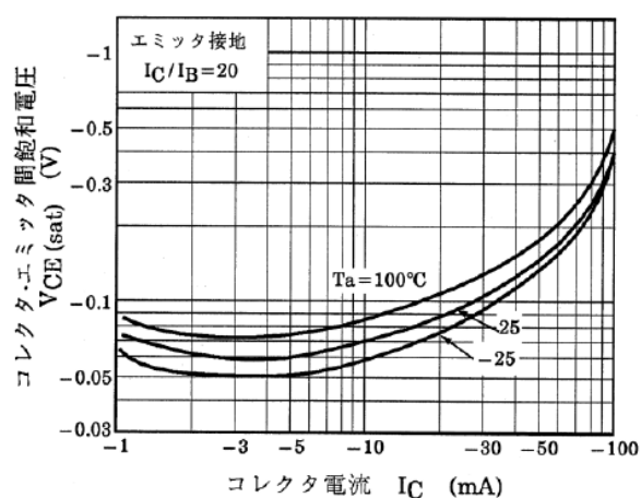
図 10.10 RN2407 V_{CE(sat)} - I_C
