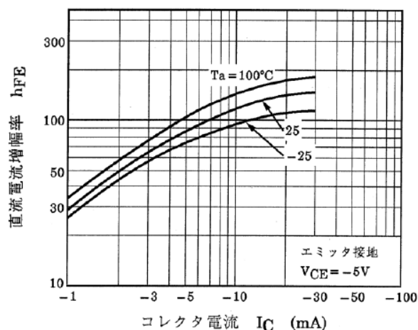
図 10.9 RN2409 h_{FE} - I_C
