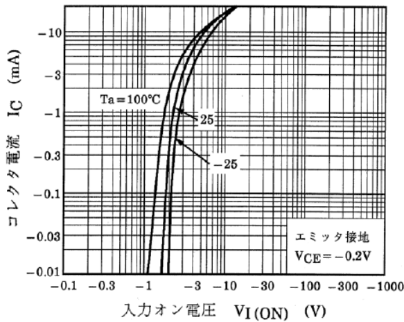
図 10.3 RN2409 I_C - V_{I(ON)}
