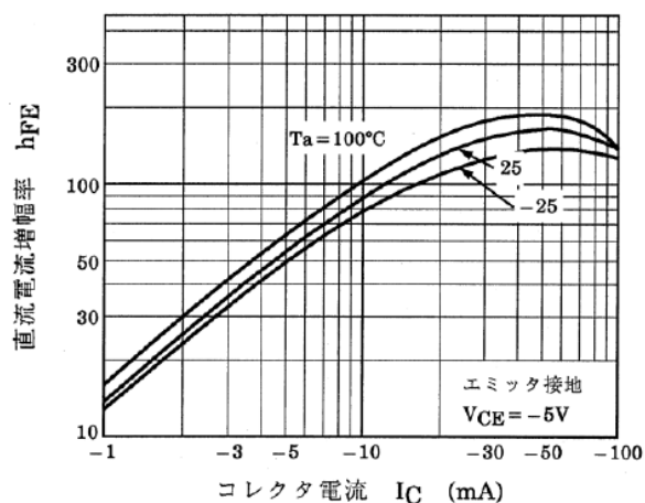
図 10.7 RN2407 h_{FE} - I_C
