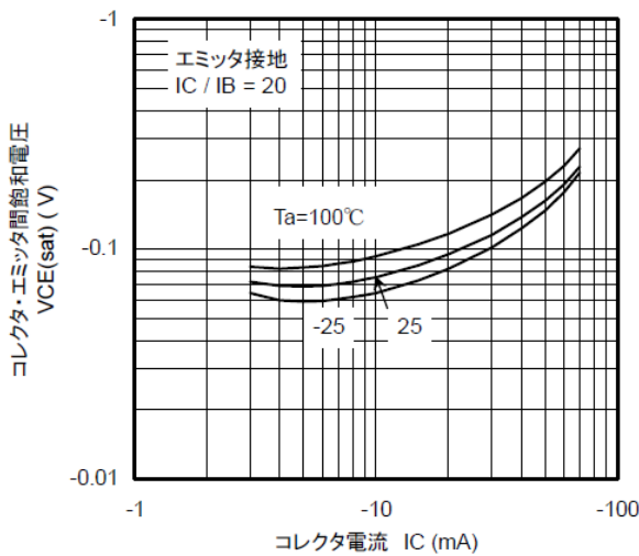
図 10.20 RN2418 V_{CE(sat)} - I_C
