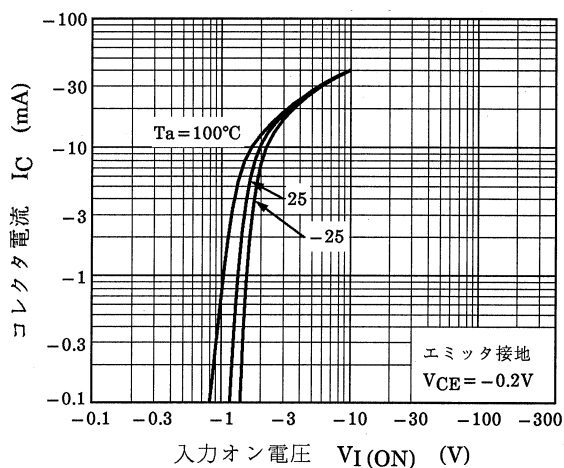
図 7.1 RN2607 I_C - V_{I(ON)}
