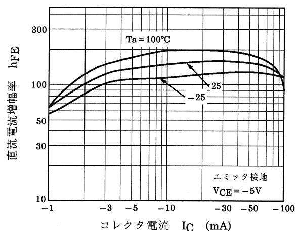
図 7.6 RN2608 h_{FE} - I_C
