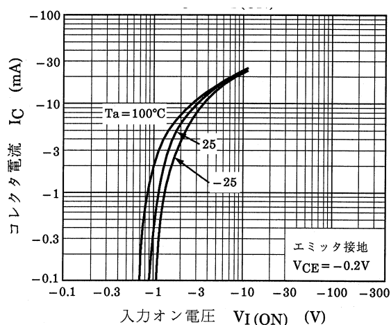
図 7.3 RN2608 I_C - V_{I(ON)}
