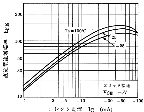
図 7.5 RN2607 h_{FE} - I_C
