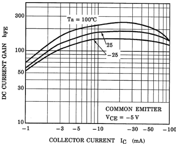
Fig. 10.17 RN2905 h_{FE-IC}
