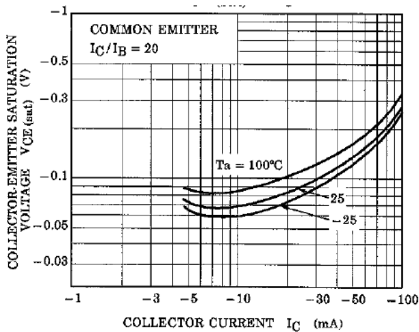
Fig. 10.19 RN2901 V_{CE(sat)}-I_C
