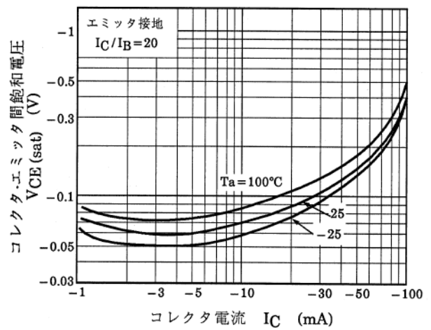
図 10.10 RN2907 V_{CE(sat)}-I_C
