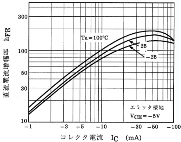
図 10.7 RN2907 h_{FE}-I_C
