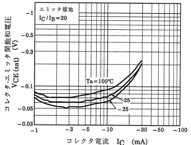
図 10.12 RN2909 V_{CE(sat)}-I_C
