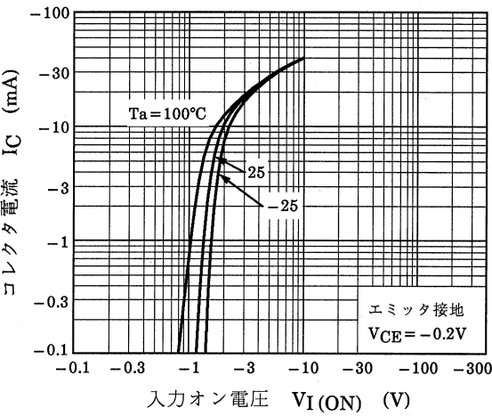
図 12.1 Q1 I_C - V_{I(ON)}
