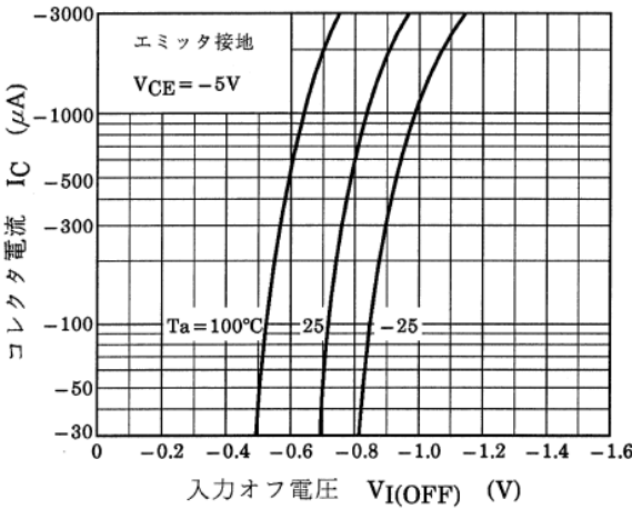
図 12.2 Q1 I_C - V_{I(OFF)}
