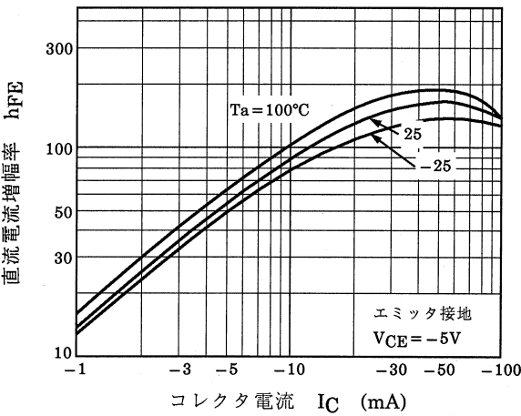
図 12.3 Q1 h_{FE} - I_C
