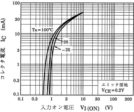
図 12.4 Q2 I_C - V_{I(ON)}
