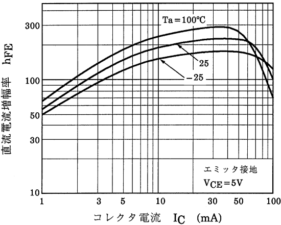
図 12.6 Q2 h_{FE} - I_C
