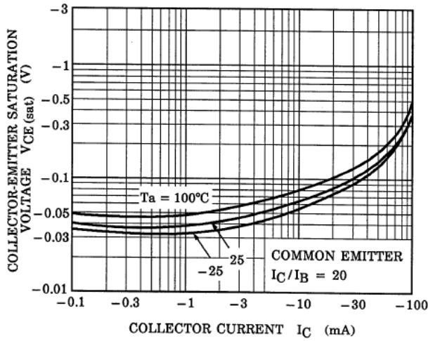
Fig. 13.7 Q1 V_{CE(sat)}-I_C
