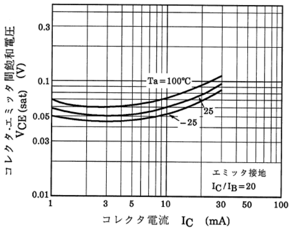
図 13.7 Q1 V_{CE(sat)}-I_C
