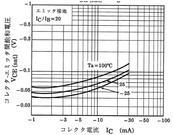
図 13.8 Q2 V_{CE(sat)}-I_C
