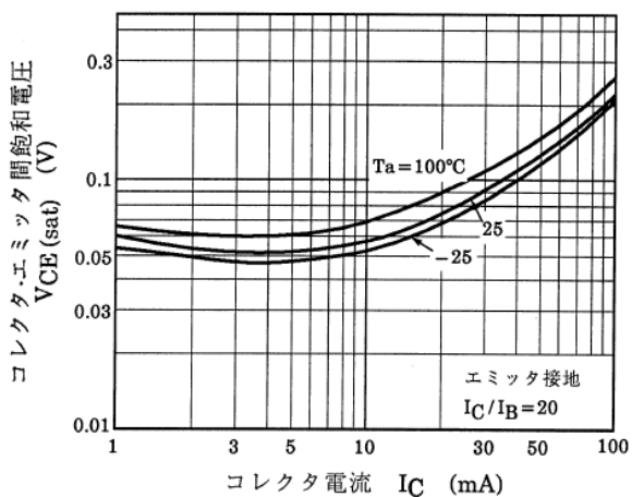
図 13.7 Q1 V_{CE(sat)}-I_C
