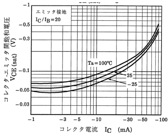
図 13.8 Q2 V_{CE(sat)}-I_C
