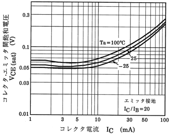
図 13.7 Q1 V_{CE(sat)}-I_C
