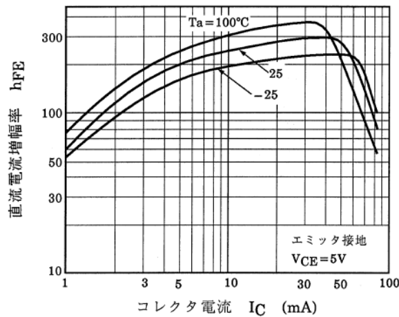
図 13.5 Q1 h_{FE} - I_C
