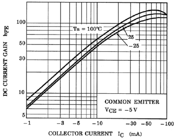
Fig. 10.13 RN2301 h_{FE}-I_C
