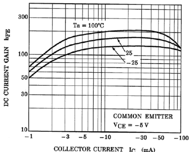
Fig. 10.18 RN2306 h_{FE}-I_C
