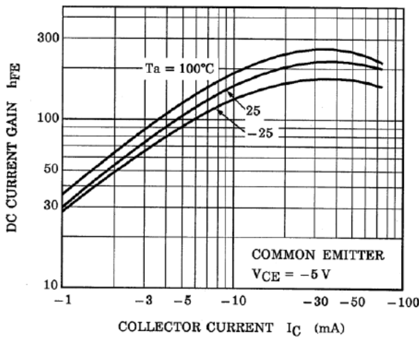
Fig. 10.15 RN2303 h_{FE}-I_C
