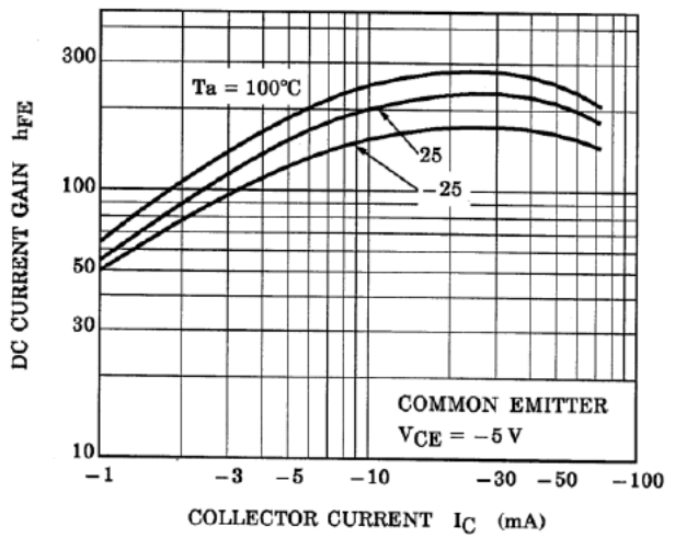
Fig. 10.16 RN2304 h_{FE}-I_C
