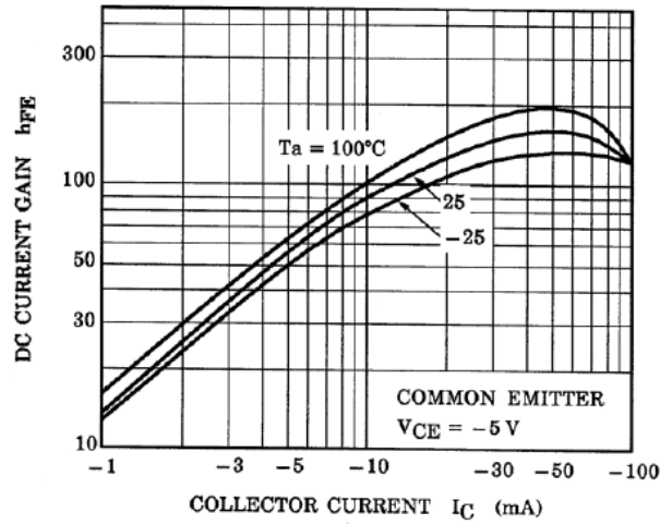
Fig. 10.14 RN2302 h_{FE}-I_C
