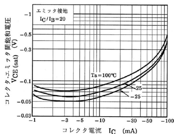
図 10.10 RN2307 V_{CE(sat)} - I_C
