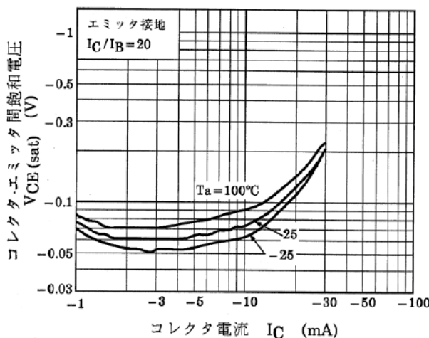
図 10.12 RN2309 V_{CE(sat)} - I_C
