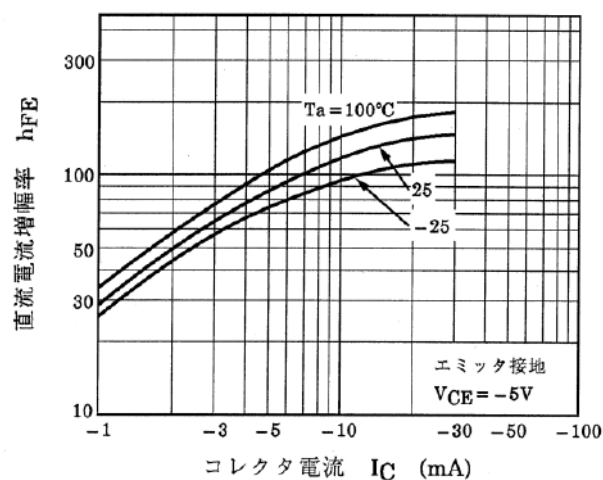
図 10.9 RN2309 h_{FE} - I_C
