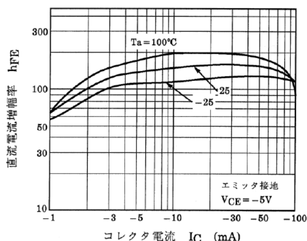
図 10.8 RN2308 h_{FE} - I_C
