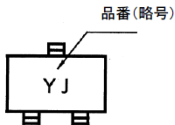
図 9.3 現品表示 RN2309
