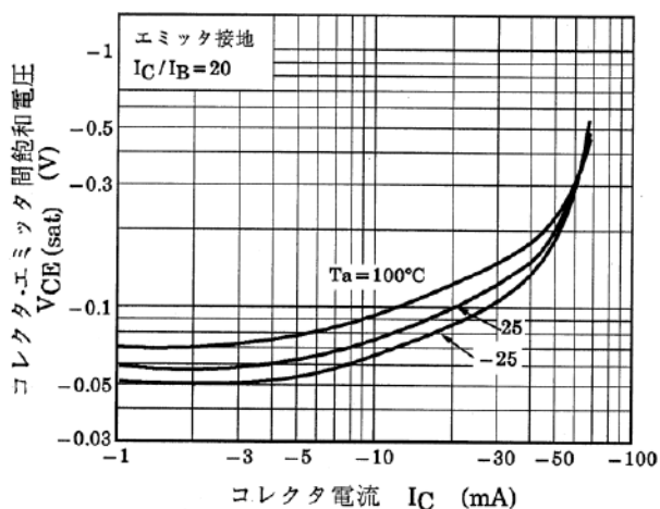
図 10.11 RN2308 V_{CE(sat)} - I_C
