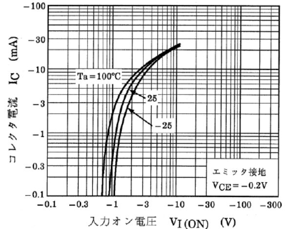
図 10.2 RN2308 I_C - V_{I(ON)}
