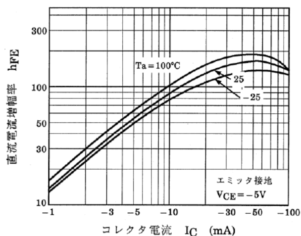
図 10.7 RN2307 h_{FE} - I_C
