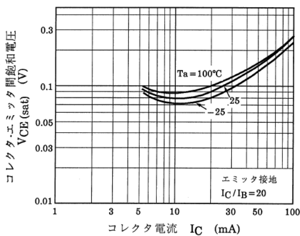
図 13.8 Q2 V_{CE(sat)}-I_C
