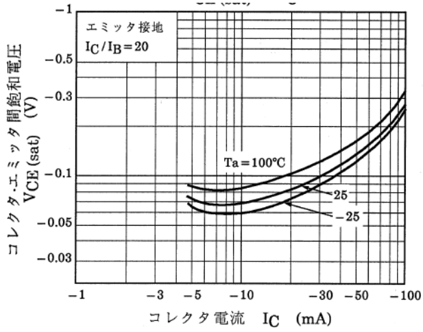
図 13.7 Q1 V_{CE(sat)}-I_C
