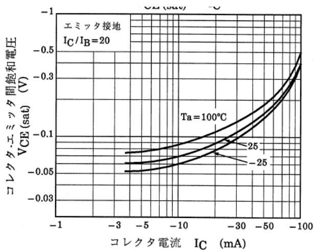
図 13.7 Q1 V_{CE(sat)}-I_C
