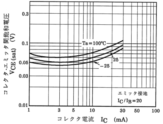
図 13.8 Q2 V_{CE(sat)}-I_C
