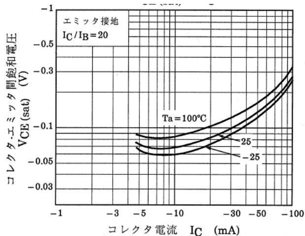
図 13.8 Q2 V_{CE(sat)}-I_C
