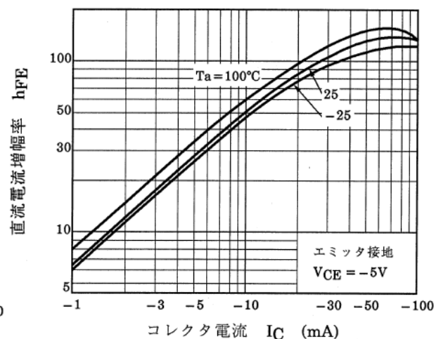
図 13.6 Q2 h_{FE} - I_C
