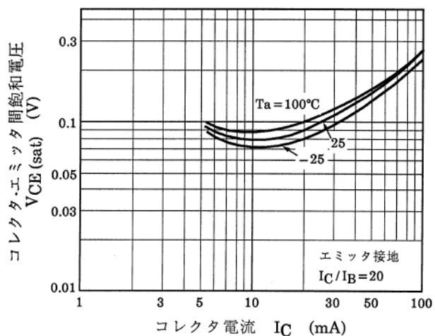
図 13.7 Q1 V_{CE(sat)}-I_C
