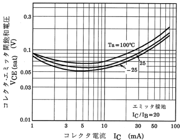
図 13.7 Q1 V_{CE(sat)}-I_C
