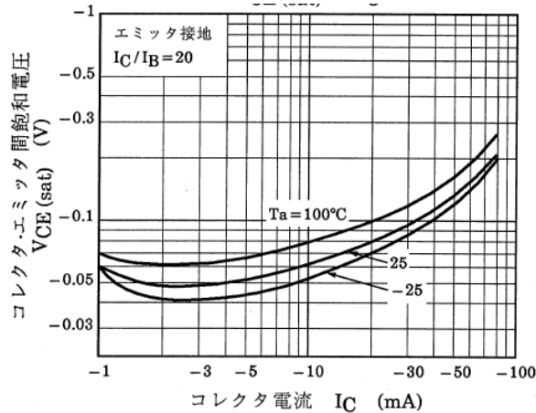
図 13.8 Q2 V_{CE(sat)}-I_C
