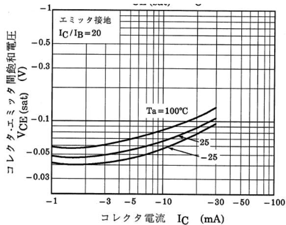
図 13.8 Q2 V_{CE(sat)}-I_C
