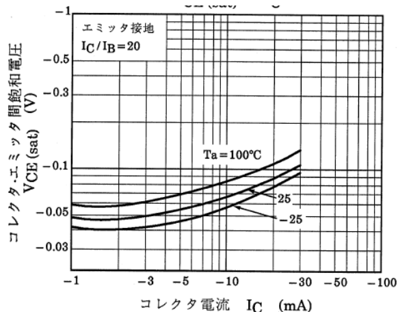
図 13.8 Q2 V_{CE(sat)}-I_C
