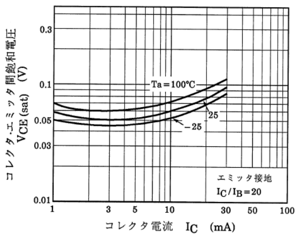
図 13.7 Q1 V_{CE(sat)}-I_C
