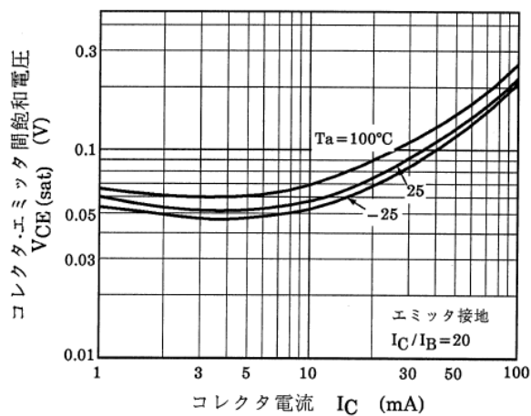
図 13.7 Q1 VCE(sat)-IC
