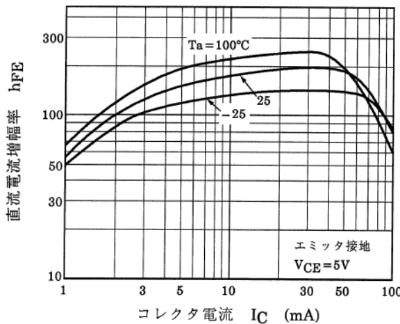
図 13.5 Q1 h_{FE} - I_C
