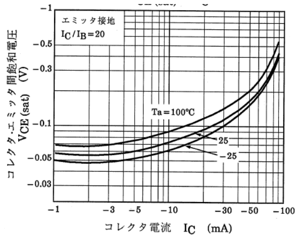
図 13.8 Q2 V_{CE(sat)}-I_C
