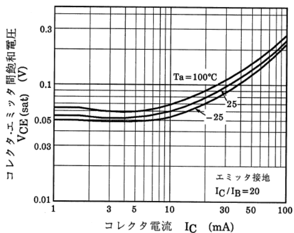
図 13.7 Q1 V_{CE(sat)}-I_C
