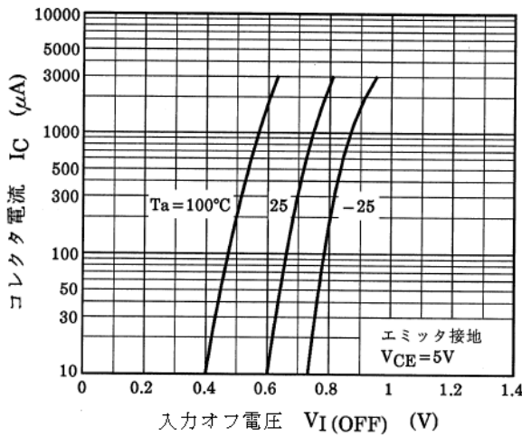
図 13.3 Q1 I_C - V_{I(OFF)}
