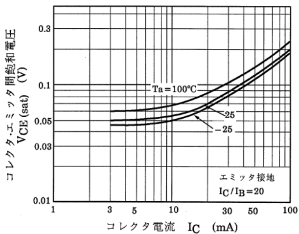
図 13.7 Q1 V_{CE(sat)}-I_C
