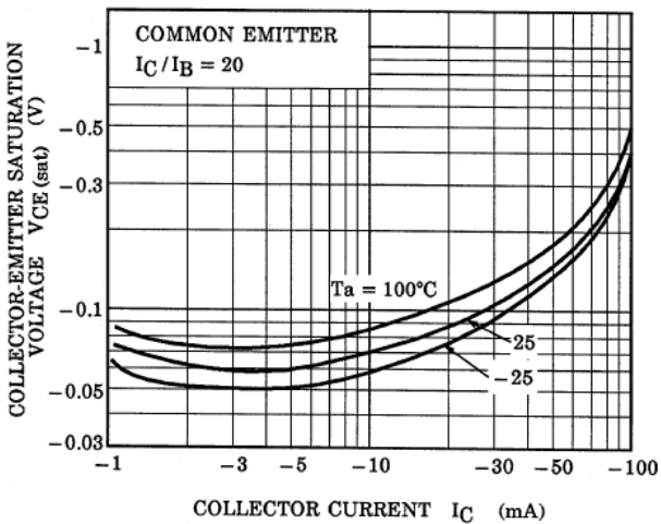
Fig. 13.8 Q2 V_{CE(sat)}-I_C
