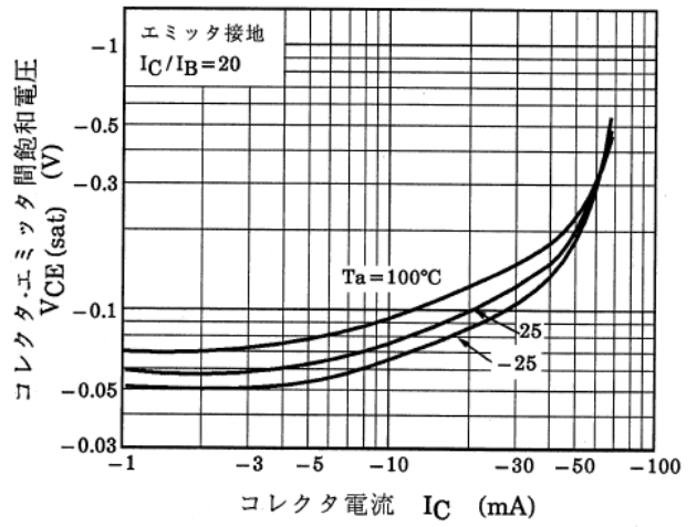
図 13.8 Q2 V_{CE(sat)}-I_C
