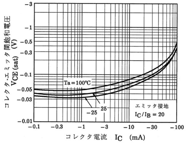
図 13.8 Q2 V_{CE(sat)}-I_C
