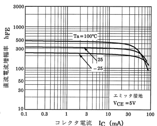
図 9.6 RN1911FE h_{FE} - I_C
