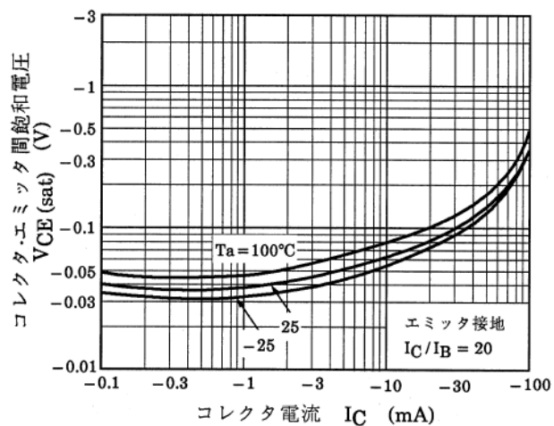
図 9.7 RN2910FE V_{CE(sat)}-I_C
