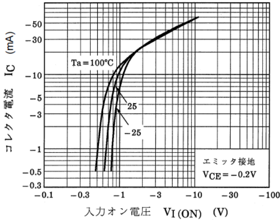
図 9.1 RN2910FE I_C - V_{I(ON)}
