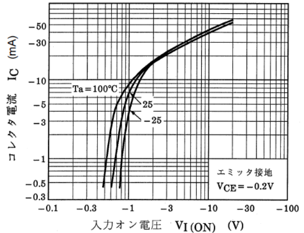
図 9.2 RN2911FE I_C - V_{I(ON)}
