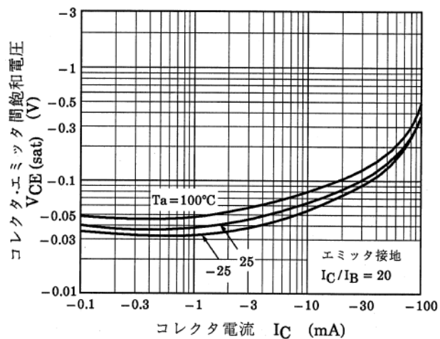
図 9.8 RN2911FE V_{CE(sat)}-I_C
